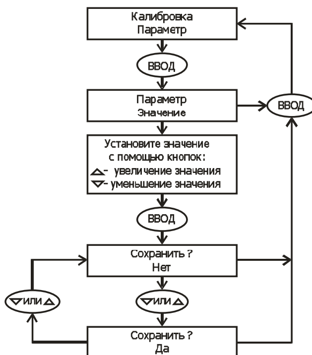
Рис. 2 – Обобщенный алгоритм ввода параметров в режиме «Калибровка» Таблица 3
