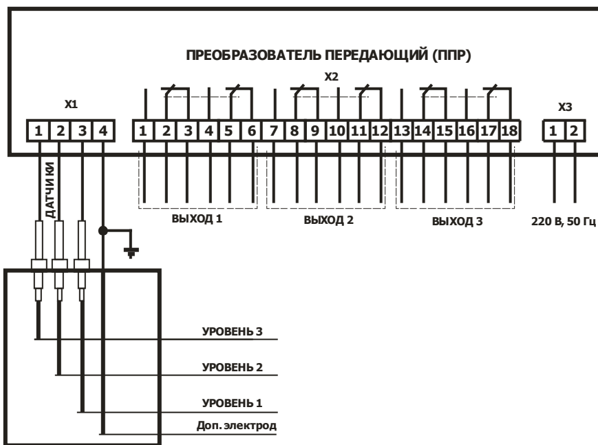
Рис. В.2 – Вариант для резервуаров из непроводящих материалов
