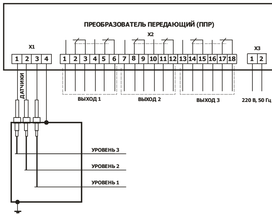
Рис. В.1 – Вариант для металлических резервуаров
