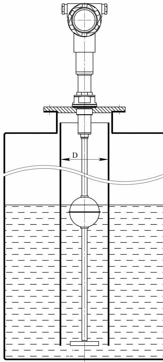
Рис. Д-2. Монтаж с грузом в успокоительной трубе. D – внутренний диаметр успокоительной трубы, мм, не менее 170
