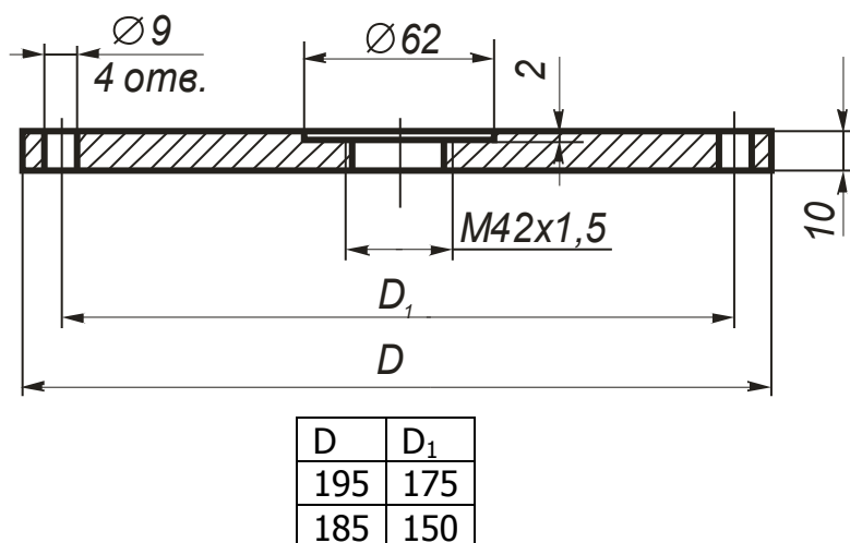
Рис. В.1 Фланец для монтажа РУПТ-М на емкость без избыточного давления
